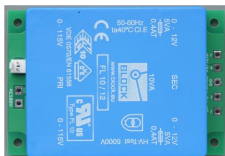
図6 トランス実装状態
