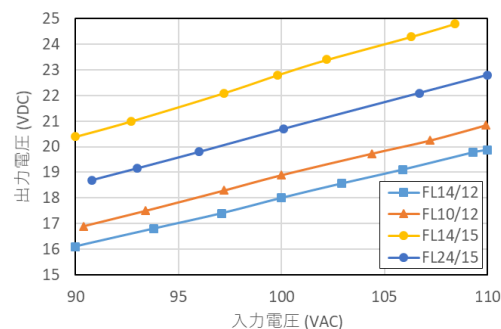
図5 電源電圧特性例
