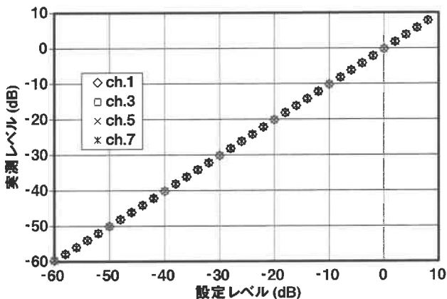
〈第6図〉 設定レベルの 実測データ
