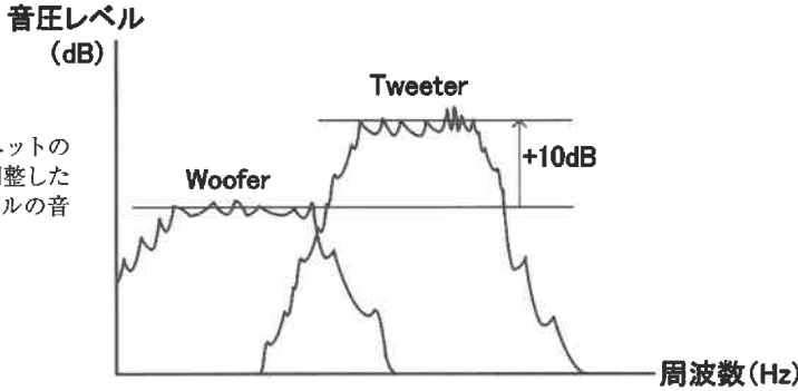
(a) 従来型のチャンネル・ディバイダでのVR調整
