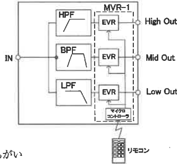
(b) MVR-1を用いたレベル調整
