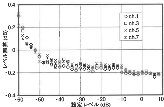
〈第7図〉 設定レベル の誤差
