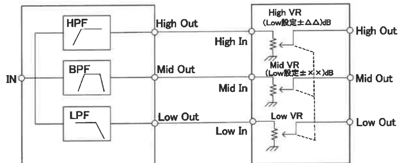
〈第1図〉本機を用いたときのチャンネル・ディバイダのレベル調整
